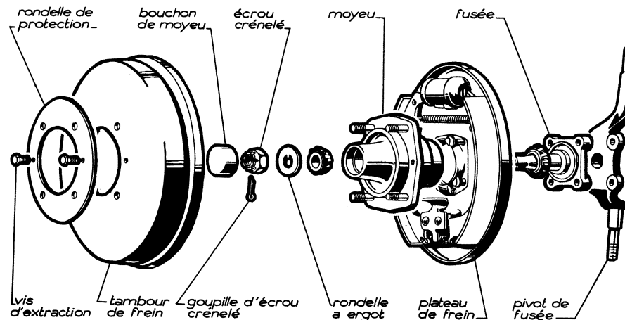
Fig. 2. - Assembly of front hub Bild 2. - Montage der Vorderradnabe
